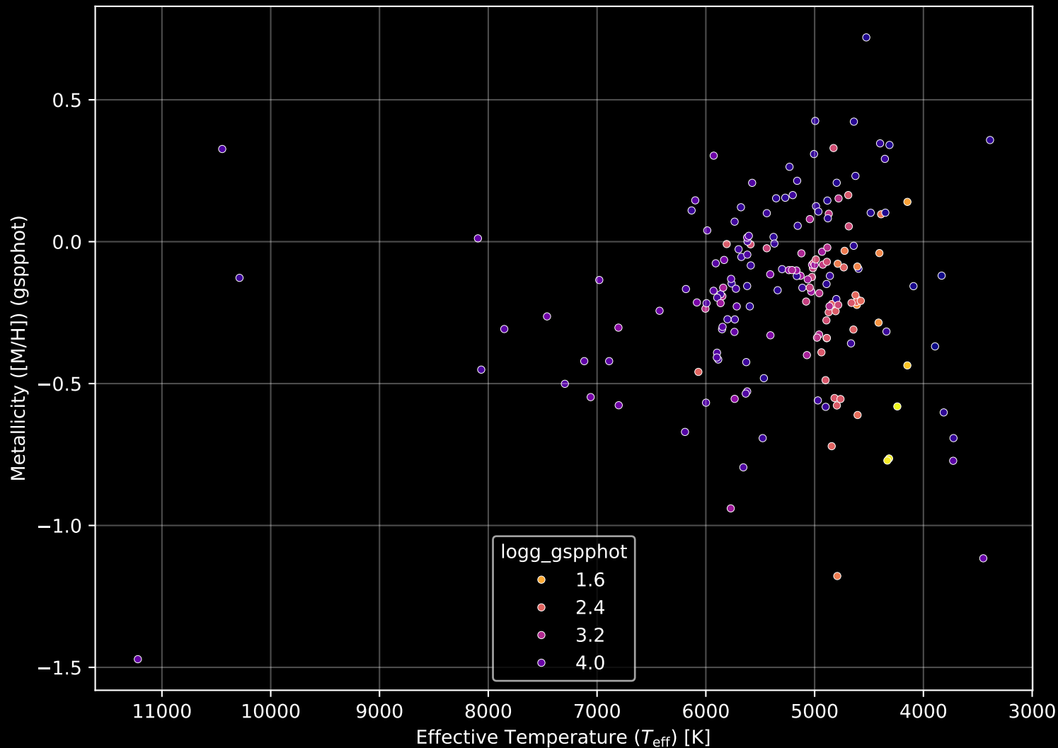
APOGEE DR17 Field: [273-28-O_TESS] Stellar Population Parameters (n= 181)
